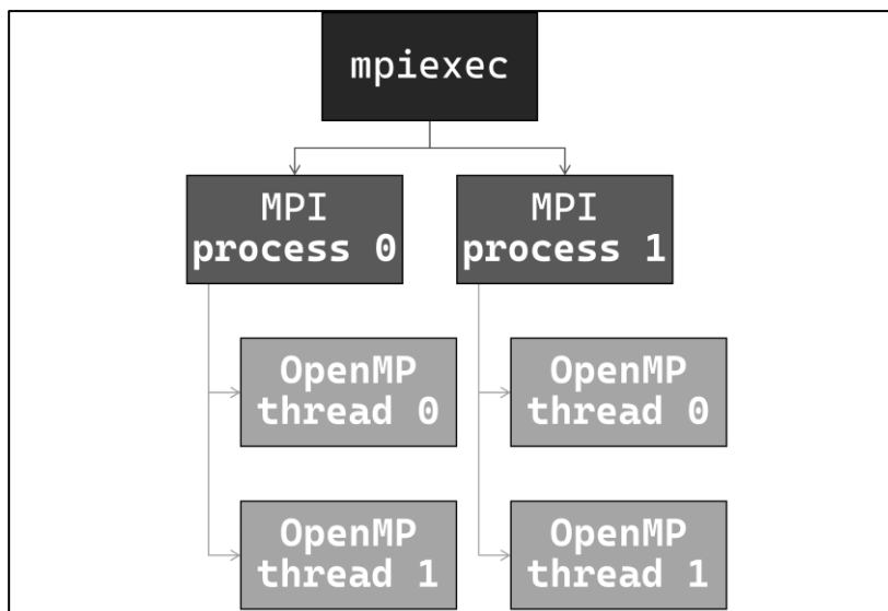
Slika 20: Shematski prikaz / stablo hibridne paralelizacije
