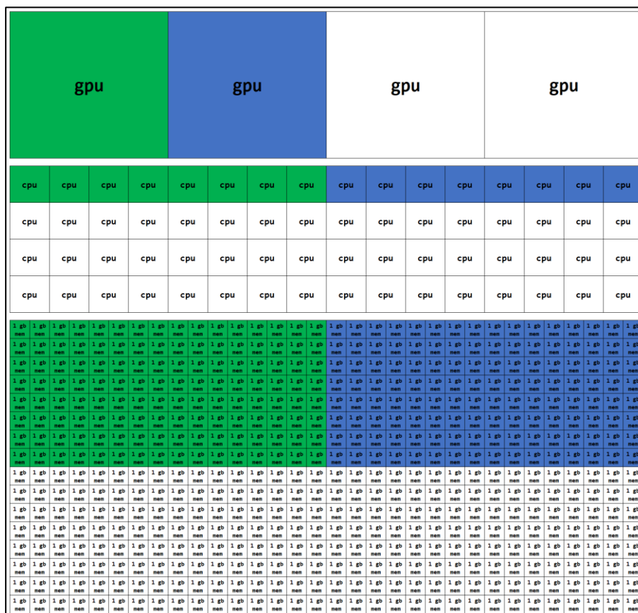
Slika 16: Raspodjela resursa za #PBS -l select=2:ngpus=1:ncpus=8:mem=128gb #PBS -l place=pack
