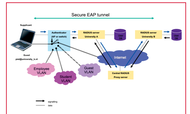
Dijagram sigurne autentikacije putem EAP tunela u bežičnoj mreži sveučilišta
